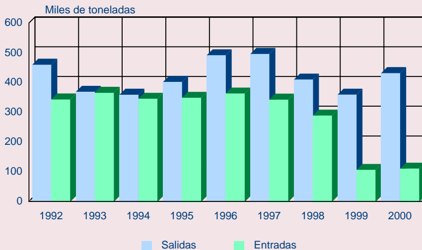
G-11.5. Evolución de las mercancías transportadas por ferrocarril. 1992-2000
